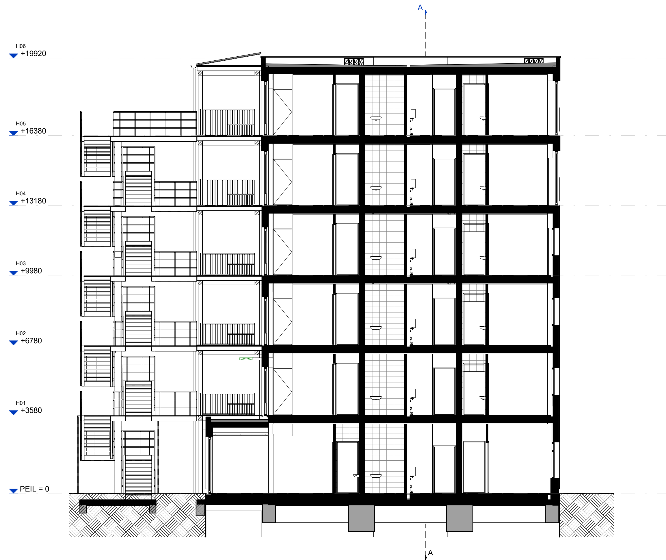
De Kapitein - Dwarsdoorsnede B SCHAAL 1 : 100
