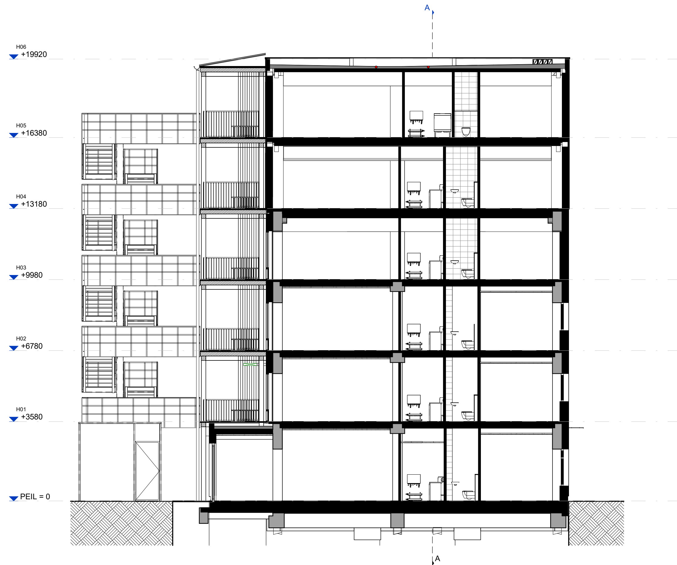
De Kaptitein - Dwarsdoorsnede C SCHAAL 1 : 100
