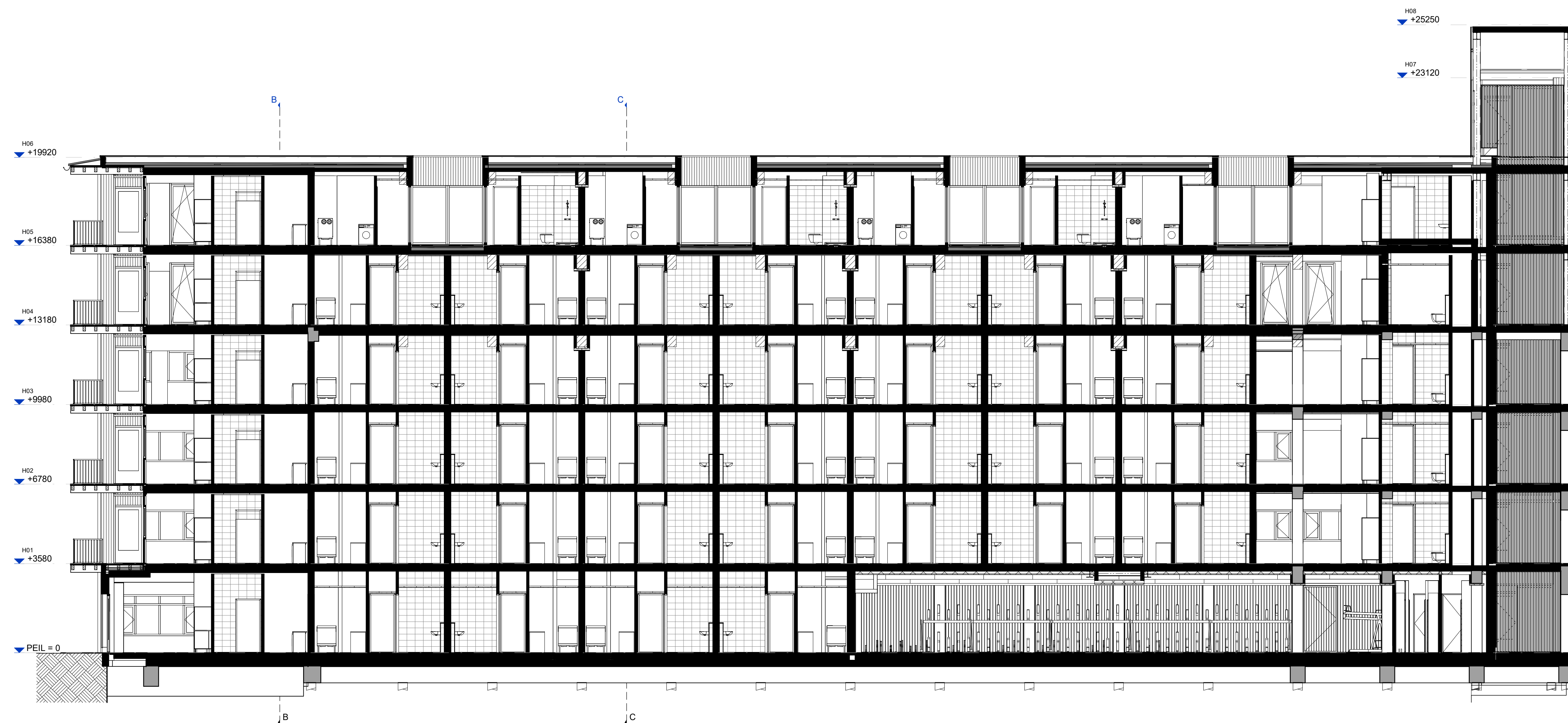
De Kapitein - Langsdoorsnede A SCHAAL 1 : 100
